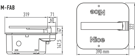
WYMIARY
