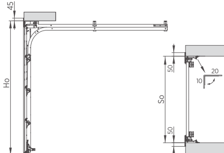
Montaż w otworze - maskownica przed otworem
